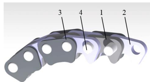
Fig. 1. Silent chain.
